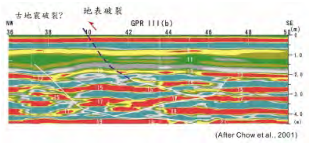
圖九 錦園地區池上斷層之透地雷達地下構造影像（依據Chow et al., 2001）。圖上顯示在處有過去斷層活動紀錄，有可能代表古地震的斷層活動。
